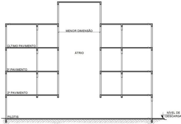
Figura 24: Modelo 1 de átrios cobertos fechados
