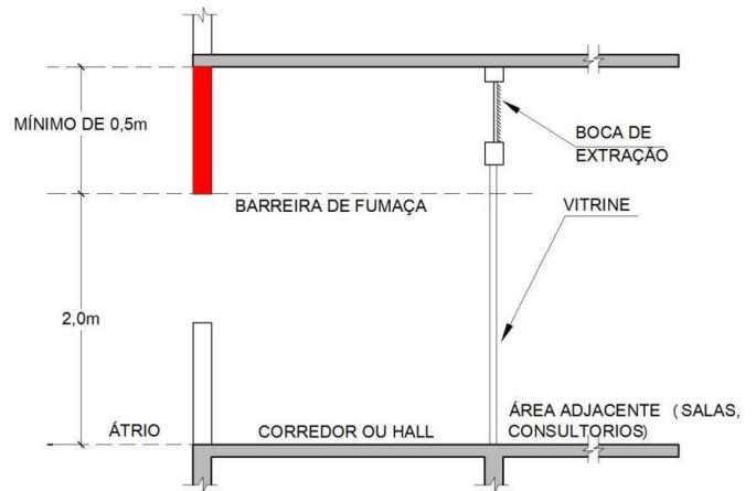
Figura 31: Exemplo de locais diretamente abertos, porém separados do átrio por uma circulação horizontal
