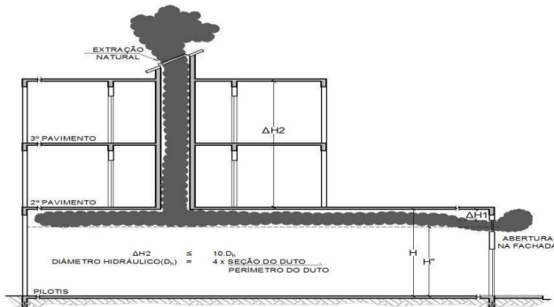
Figura 8: Diâmetro hidráulico
