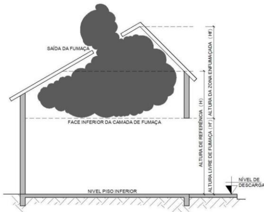
Figura 3: Altura de referência, altura livre de fumaça e zona enfumaçada
