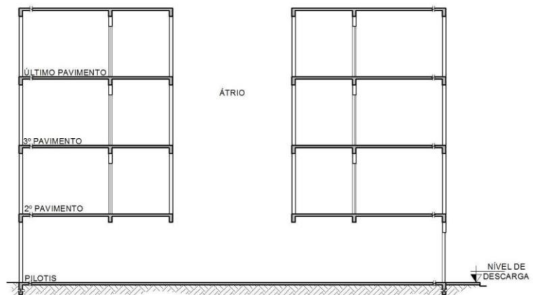
Figura 22: Átrio ao ar livre
