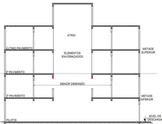
Figura 29: Fechamento do átrio
