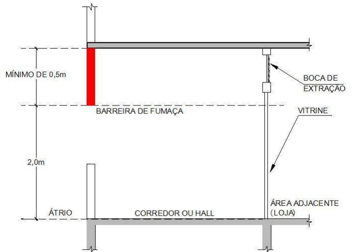
Figura 4: Detalhe de barreira de fumaça – corte
