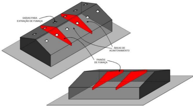
Figura 2: Elementos do sistema de controle de fumaça
