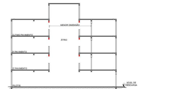
Figura 23: Átrio coberto aberto
