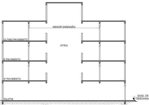
Figura 25: Modelo 2 de átrios cobertos fechados
