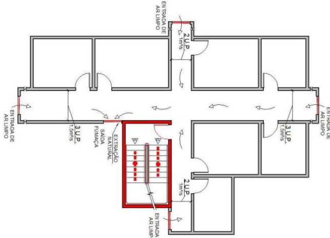
Figura 20: Rotas de fuga com largura variável
