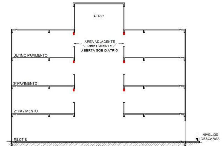
Figura 32: Exemplo de locais diretamente abertos sob o átrio
