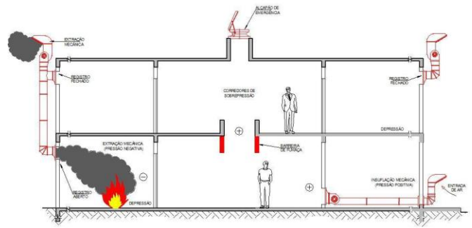
Figura 21: Controle por sobrepressão
