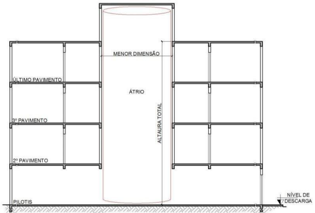
Figura 27: Dados relativos a um átrio coberto padronizado
