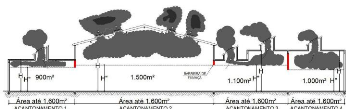
Figura 6: Altura de referência diversificada por acantonamento
