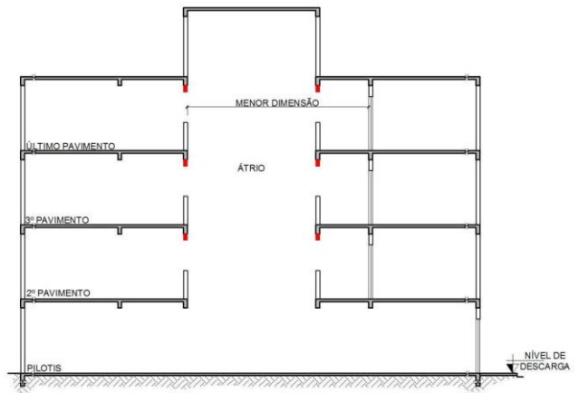
Figura 26: Átrio considerado aberto de um lado e fechado do outro
