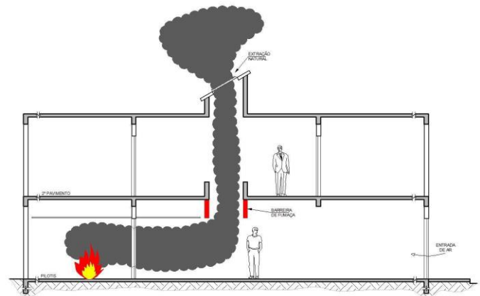
Figura 11: Exemplo de controle de fumaça natural
