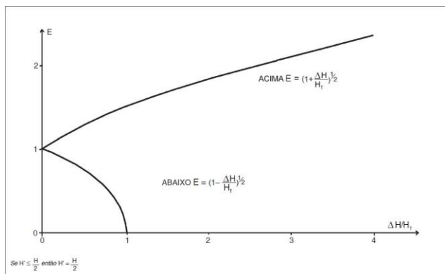
Figura 7 - Eficiência dos Exaustores
