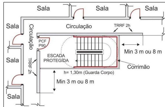
Figura 13 - Escada aberta externa
