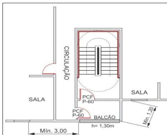
Figura 10 - Escada enclausurada do tipo PF ventilada por balcão
