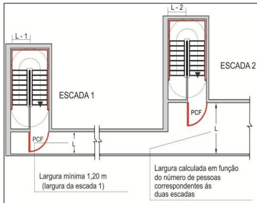
Figura 19 – Dimensionamento de corredores de descarga
