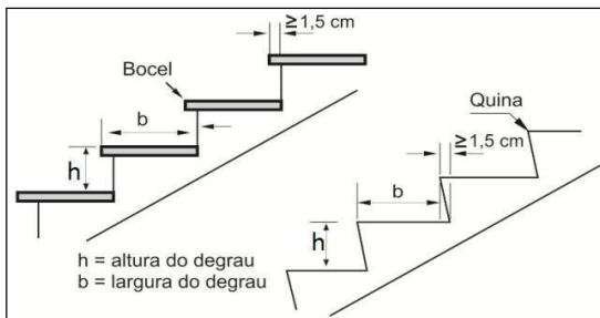
Figura 4 - Altura e largura dos degraus
