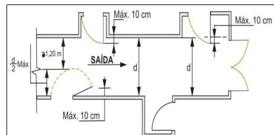
Figura 2 - Abertura das portas no sentido de saída
