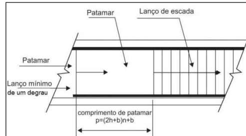
Figura 5 - Lanço mínimo e comprimento de patamar
