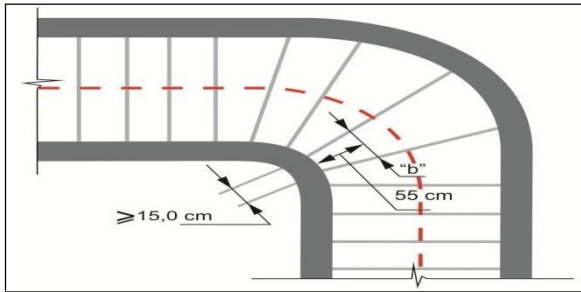
Figura 6 - Escada com lanços curvos e degraus balanceados
