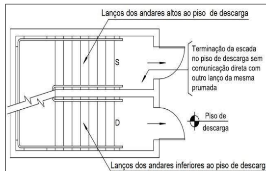
Figura 3 - Segmentação das escadas no piso da descarga
