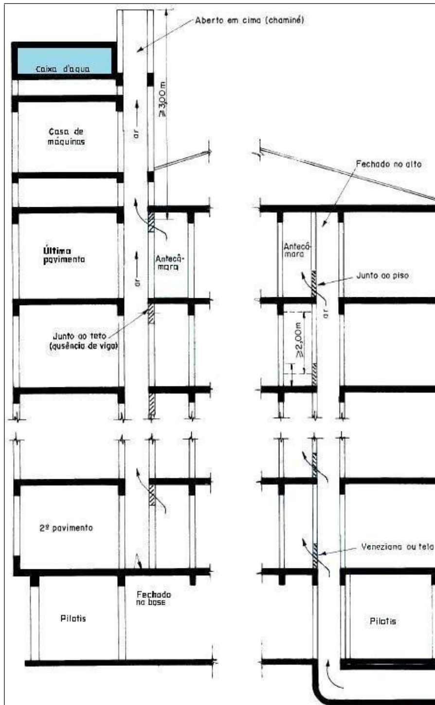
Figura 11 - Exemplo de dutos de ventilação (corte AB e corte CD)
