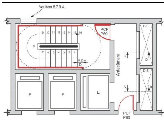
Figura 9 - Escada enclausurada à prova de fumaça
